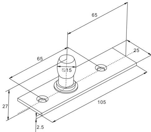
Pivot mobile à montage en surface Code No.: CDPH008
