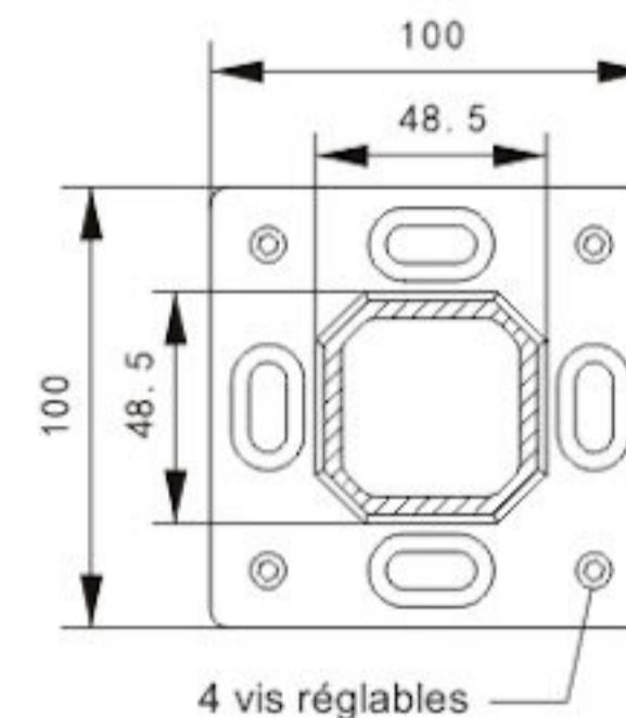
Installation au plancher:
