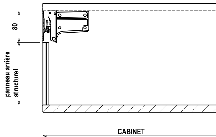
VUE LATÉRALE
