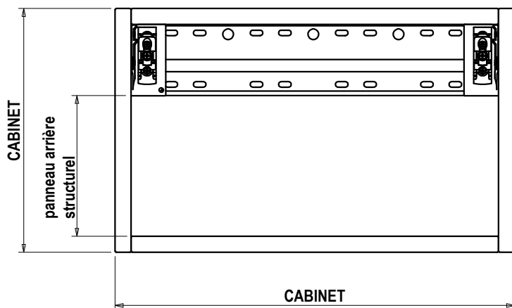
VUE FRONTALE
