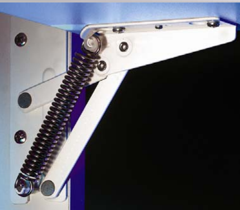
542L30 – Charnière à ressort côté gauche
