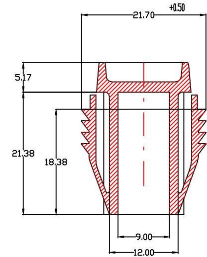
View A-B
