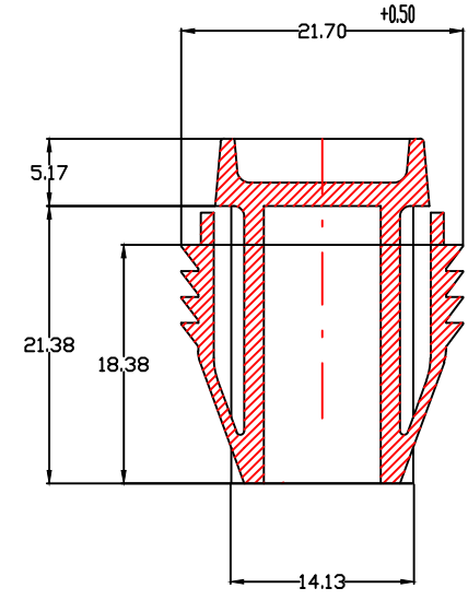
View A-B
