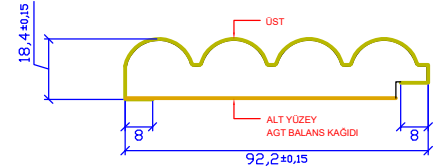
HG FOLYO KAPLANMIŞ GÖRÜNÜM HG FOIL COATING VIEW ЧЕРТЕЖ КАДЕТРИ С ТИВХ ПАМІНІРОВАНИЕМ ПОКРЫТИЕМ مطابق عرض رافانقي بي سي سي مطبوع تصوير افراز شده فویل بی سی سی HG FOIL VUE DE FOIL FRAISE
