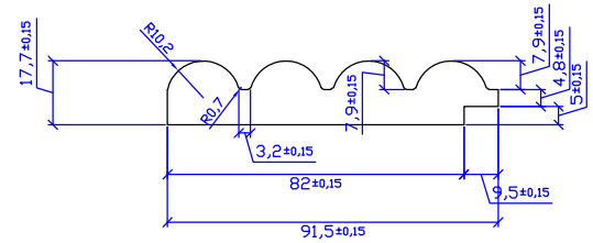
HG FOLYO FREZELENMİŞ GÖRÜNÜM MILLED HG FOLIO VIEW ЧЕРТЕЖ КАДЕТРИ С ТИВХ ПАМІНІРОВАНИЕМ И ФРЕЗЕРНОЙ ОБРАБОТКОЙ عرض رافانقي بي سي سي مطبوع تصوير افراز شده فویل بی سی سی HG FOIL VUE DE FOIL FRAISE
