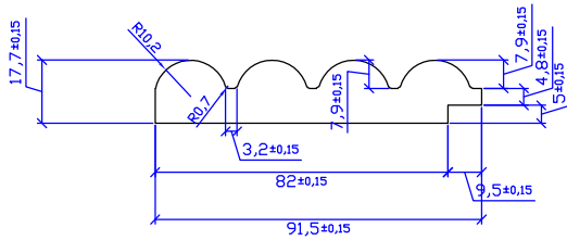
PVC FOLYO FREZELENMİŞ GÖRÜNÜM MILLED PVC FOIL VIEW ЧЕРТЕЖ КАДЕТРИ С ТИВХ ПАМІНІРОВАНИЕМ И ФРЕЗЕРНОЙ ОБРАБОТКОЙ عرض رافانقي بي سي سي مطبوع تصوير افراز شده فویل بی سی سی PVC FOIL PERSPECTIVES face
