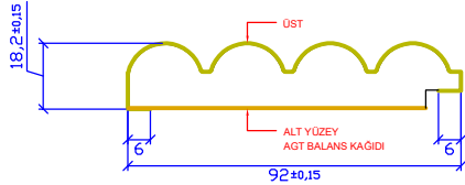
PVC FOLYO KAPLANMIŞ GÖRÜNÜM PVC FOIL COATING VIEW ЧЕРТЕЖ КАДЕТРИ С ТИВХ ПАМІНІРОВАНИЕМ ПОКРЫТИЕМ عرض رافانقي بي سي سي مطبوع تصوير افراز شده فویل بی سی سی PVC FOIL PERSPECTIVES COUVERTURE face
