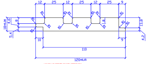
HG FOLYO FREZELENMİŞ GÖRÜNÜM MILLED HG FOIL VIEW ЧЕРТЕЖ ИЗДЕЛИЯ С ПГНЦЕВЫМ ЛАМИНИРОВАНИЕМ И ФРЕЗЕРНОЙ ОБРАБОТКОЙ مطابق: هوزان شنه فويل سي اسي سي تصميم: هوزان شنه فويل سي وي سي HG FOIL VUE DE FOIL FRAISE
