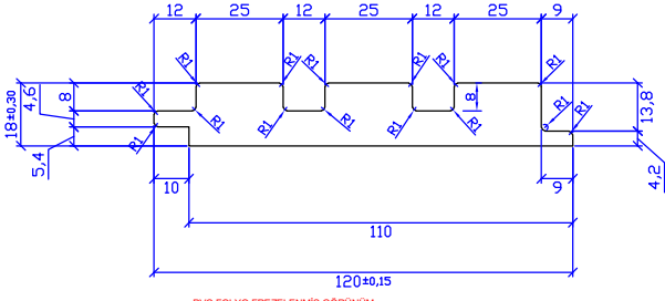
PVC FOLYO FREZELENMİŞ GÖRÜNÜM MILLED PVC FOIL VIEW ЧЕРТЕЖ ИЗДЕЛИЯ С ПВХ ЛАМИНИРОВАНИЕМ И ФРЕЗЕРНОЙ ОБРАБОТКОЙ عروض رشاقتي سي اسي سي مكنون تصميم: هوزان شنه فويل سي وي سي PVC FOIL PERSPECTIVES fraise
