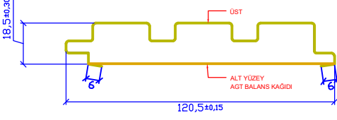
PVC FOLYO KAPLANMIŞ GÖRÜNÜM PVC FOIL COATING VIEW ЧЕРТЕЖ ИЗДЕЛИЯ С ПВХ ЛАМИНИРОВАНЫМ ПОКРЫТИЕМ عروض رشاقتي سي اسي سي مطبق تصميم: هوزان شنه فويل سي وي سي PVC FOIL PERSPECTIVES COUVERTURE fraise
