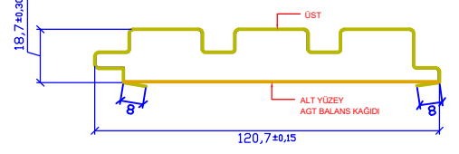
HG FOLYO KAPLANMIŞ GÖRÜNÜM HG FOIL COATING VIEW ЧЕРТЕЖ ИЗДЕЛИЯ С ПГНЦЕВЫМ ЛАМИНИРОВАНЫМ ПОКРЫТИЕМ مطابق: هوزان شنه فويل سي اسي سي تصميم: هوزان شنه فويل سي وي سي HG FOIL VUE DE FOIL FRAISE
