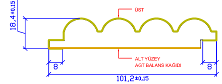
HG FOLYO KAPLANMIŞ GÖRÜNÜM HG FOIL COATING VIEW ЧЕРТЕЖ КАДЕТРИ С ТИХ ПАМІНІРОВАНИЕМ ПОКРЫТИЕМ مغطى رافقاني سي في سي تصميم اورژانده فويل سي في سي HG FOIL VUE DE FOIL FRAISE
