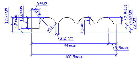
HG FOLYO FREZELENMİŞ GÖRÜNÜM MILLED HG FOIL VIEW ЧЕРТЕЖ КАДЕТРИ С ТИХ ПАМІНІРОВАНИЕМ И ФРЕЗЕРНОЙ ОБРАБОТКОЙ عرض رافقاني سي في سي مملوح تصميم اورژانده فويل سي في سي HG FOIL VUE DE FOIL FRAISE
