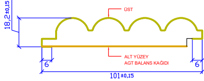
PVC FOLYO KAPLANMIŞ GÖRÜNÜM PVC FOIL COATING VIEW ЧЕРТЕЖ КАДЕТРИ С ТИХ ПАМІНІРОВАНИЕМ ПОКРЫТИЕМ عرض رافقاني سي في سي مغطى تصميم اورژانده فويل سي في سي PVC FOIL PERSPECTIVES COUVERTURE kapa
