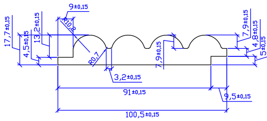
PVC FOLYO FREZELENMİŞ GÖRÜNÜM MILLED PVC FOIL VIEW ЧЕРТЕЖ КАДЕТРИ С ТИХ ПАМІНІРОВАНИЕМ И ФРЕЗЕРНОЙ ОБРАБОТКОЙ عرض رافقاني سي في سي مملوح تصميم اورژانده فويل سي في سي PVC FOIL PERSPECTIVES milled
