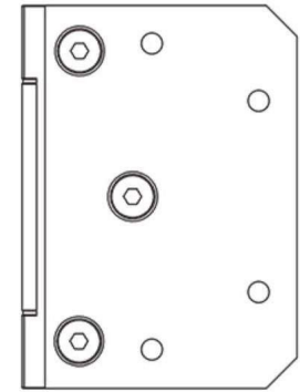
Plaque de montage
