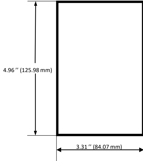
SSSM4ENDCAP2XXX
