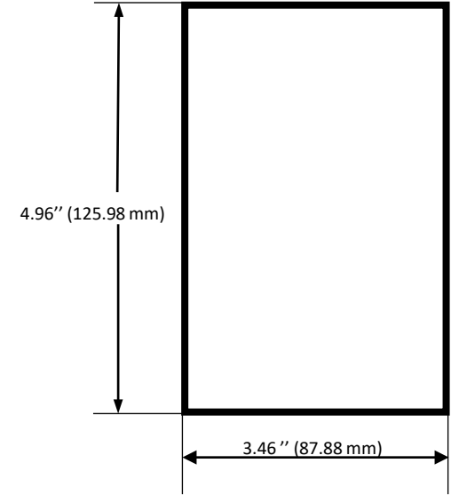
SSSM5ENDCAPXXXX
