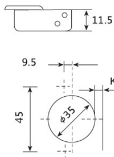
À visser/Screw-In
