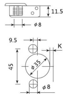
Goujon/Dowel
