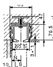
HAWA-Adapto 120
