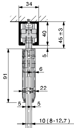
HAWA-Junior 80/GP
