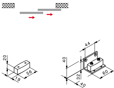
Guías inferiores puntuales.
