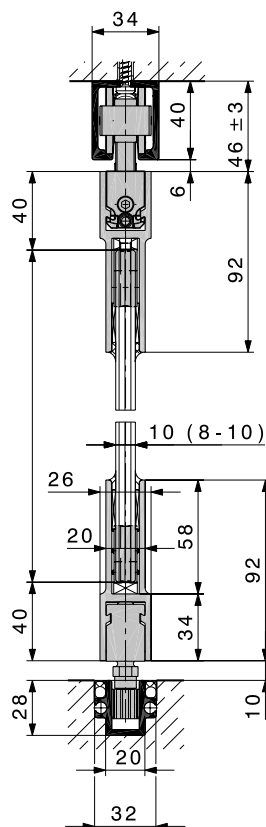
HAWA-Junior 80/G
