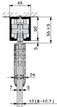
HAWA-Junior 120/GP
