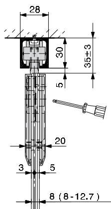
HAWA-Junior 40/GP
