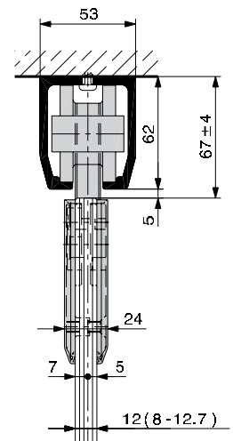
HAWA-Junior 160/GP
