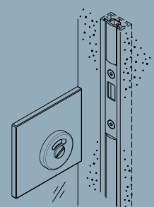
Variante cuadrada (roseta a suministrar por el cliente).
