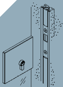
Perfil de tope mural con placa de cierre integrada.
