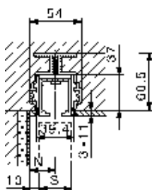
HAWA-Adapto 80
