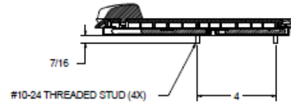
SECTION A-A
