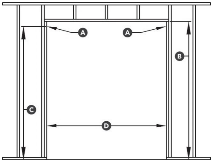
Height of Rough Opening (Table 1) | Hauteur de la baie de porte brute (Tableau 1) | Altura de la abertura en bruto (Tabla 1)
